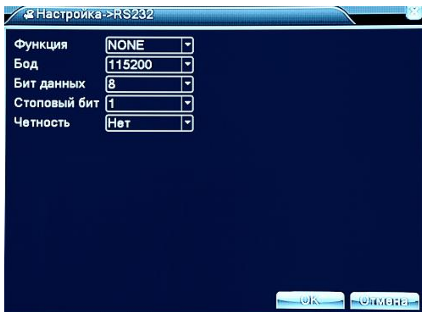
Рис. 4.30 Настройка RS232
